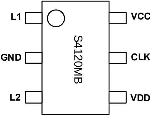
图 2 管脚封装图
